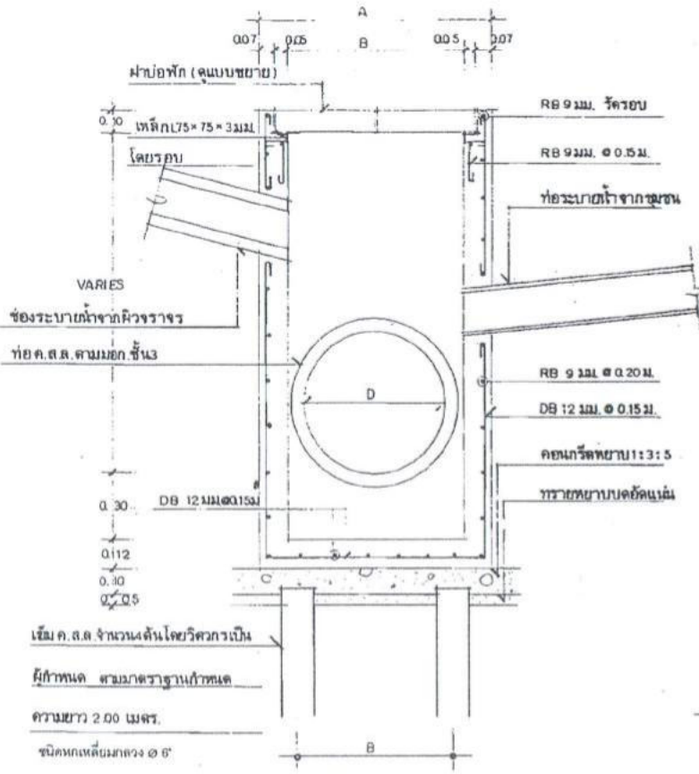
รูปตัด 2 มาตราส่วน 1:20
