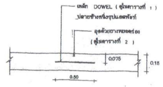
CONTRACTION JOINT NOT TO SCALE ทุกระยะไม่เกิน 10 ม.
