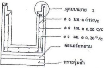
รูปตัด ①-① 1:20
