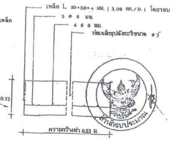
รูปตัดผ่าปอพัก 1:7.5
