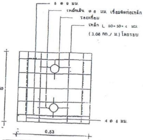
ขยายเหล็กสำหรับราง 1:7.5
