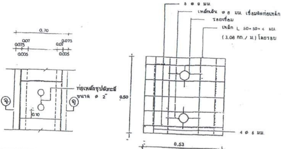
แปลนรางระบายน้ำรูปตัวยู ค.ส.ด 1:20
