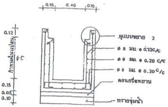
รูปตัด จ-จ 1:20
