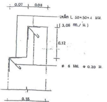
แบบขยาย ② 1:5
